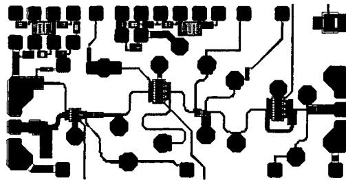
Fig. 8. LNA MMIC layout.
